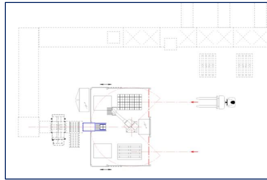
Palettisation de paquets Sorties de rotatives, façonnage
