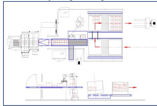
Ligne d'encaissage-palettisation Façonnage, routage
