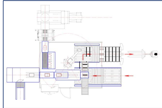
Système de mise en carton et de palettisation Sorties de rotatives, façonnage, conditionnement
